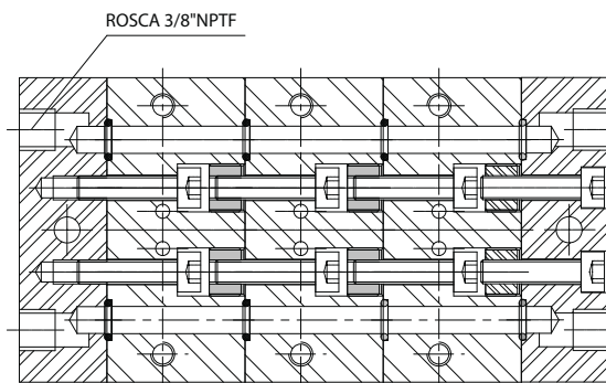
PLACA BASE
